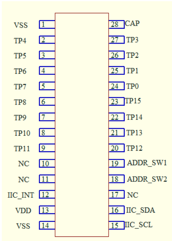
SSOP28
