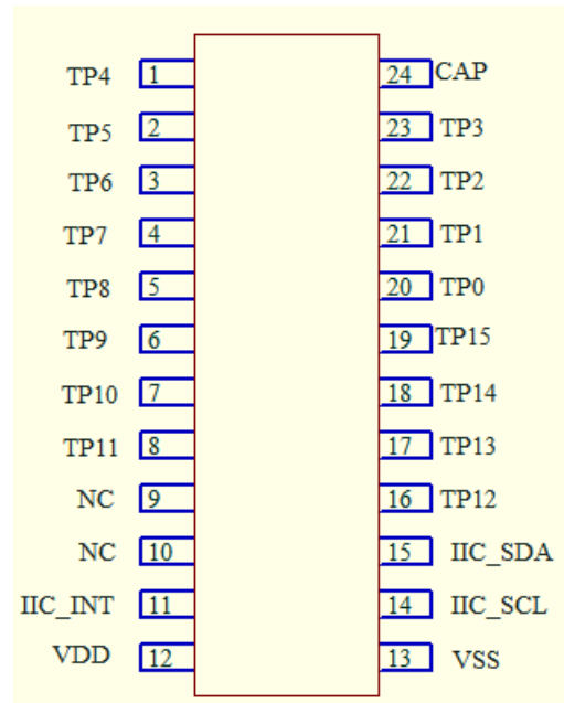
SSOP24
